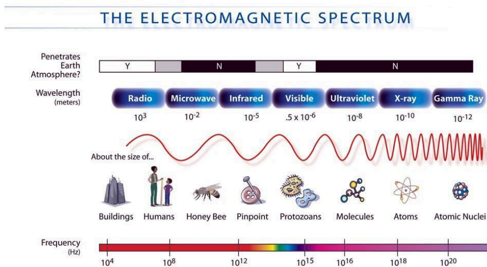
Figura 1. El espectro electromagnético. El espectro electromagnético. Las ondas electromagnéticas se clasifican en función de su longitud de onda: Ondas de radio, microondas, infrarrojos, visible, ultravioleta, rayos X y rayos gamma. Estos rayos tienen propiedades diferentes en cuanto a su tamaño,
